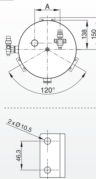
A-A Fußbild (Ausschnitt) View feet (detail)
